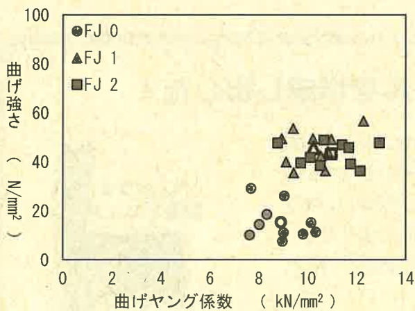
図2 炭素繊維で補強したラミナの曲げ強度性能 (●▲■：測定値、○△□：平均値)
